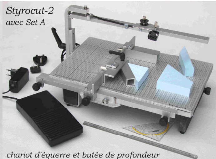
Styrocut-2
